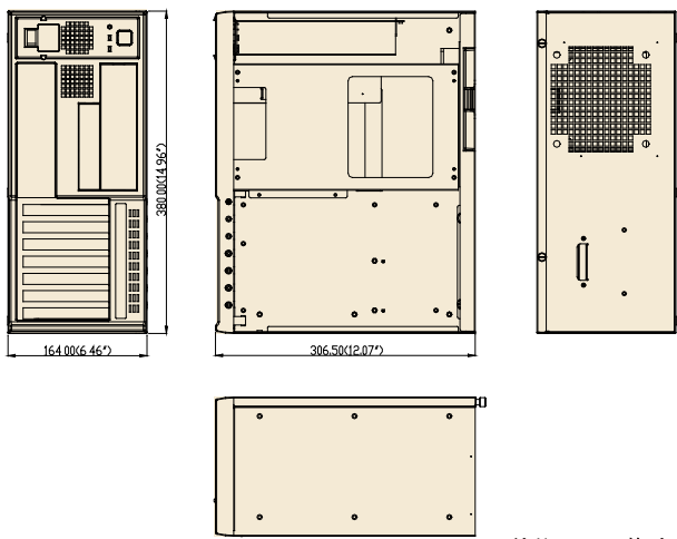
单位: mm (英寸)
