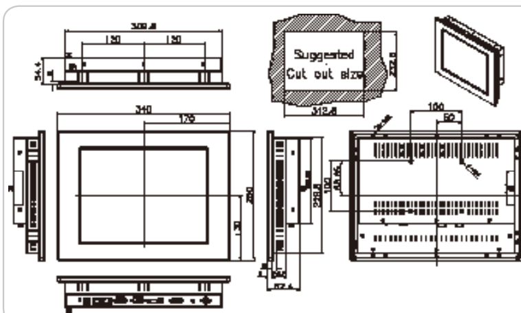
PPC-2712GS 尺寸 (单位: mm)
